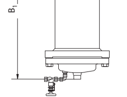
VFG2, VFGS2 D_y = 150-250 мм с удлиненным штоком для T > 140 °C
